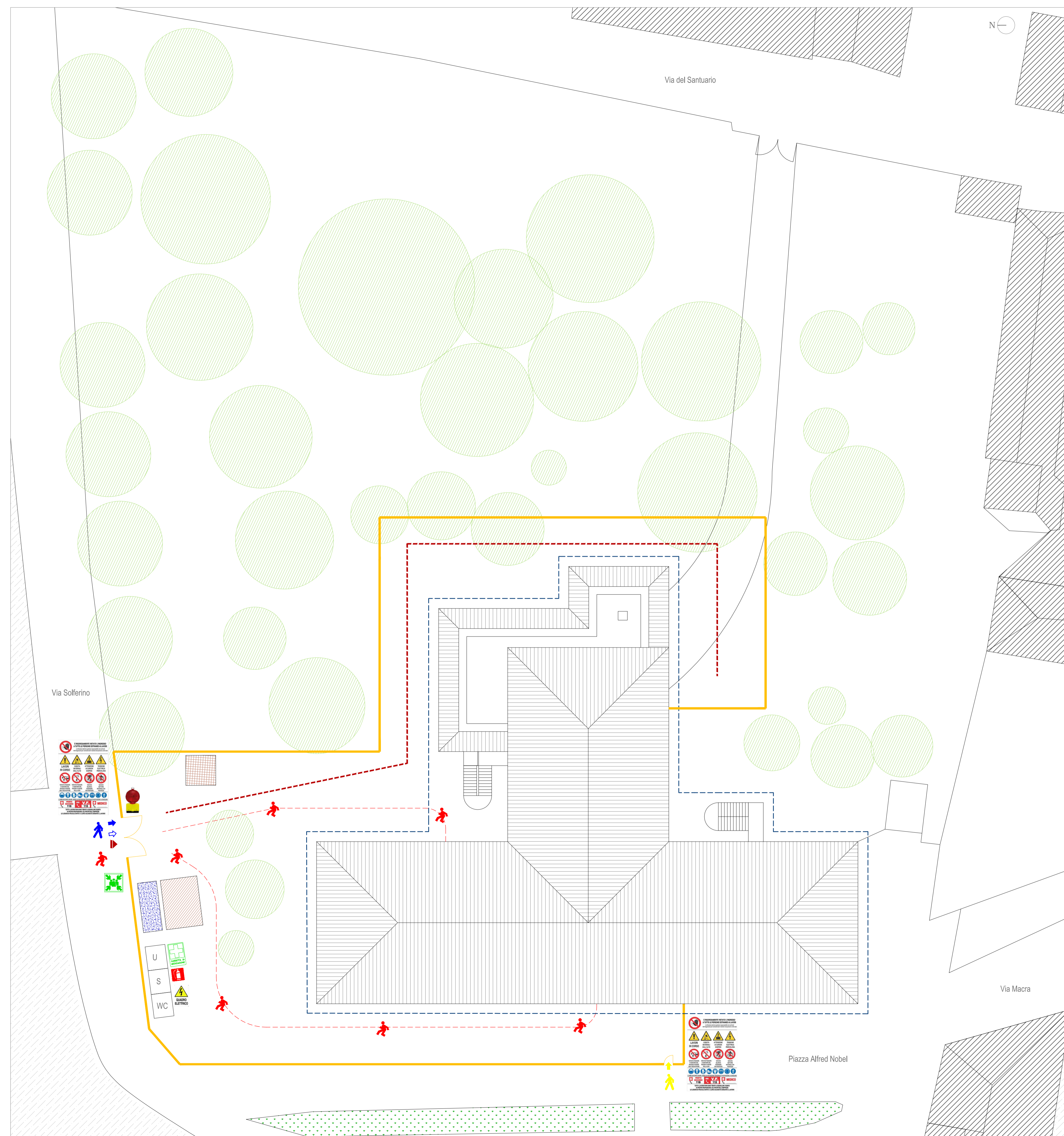
Planimetria di cantiere - scala 1:200
